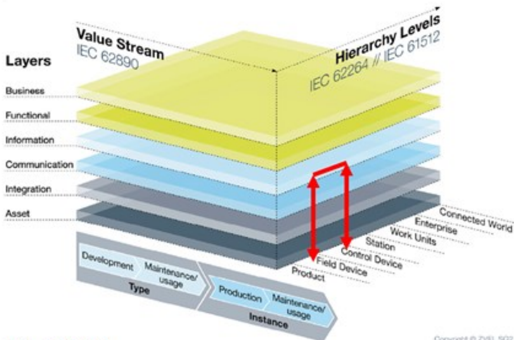
Abb. 2: RAMI 4.0
